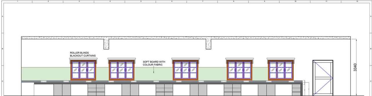
ELEVATION 1
