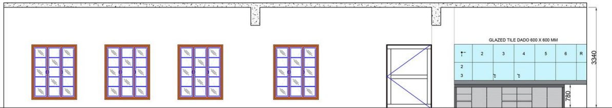
ELEVATION 2
