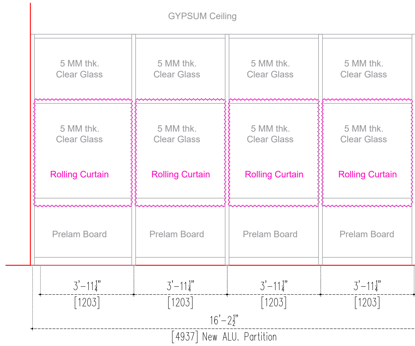
ELEVATION WALL- E
